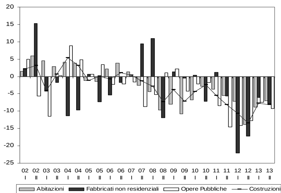
Fig. 2 – Investimenti in Costruzioni per comparto nelle Marche Variazioni percentuali in quantità rispetto all'anno precedente.
